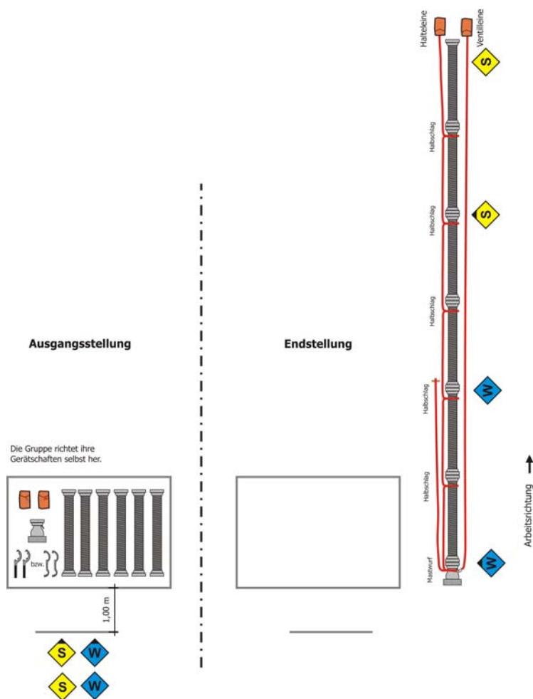
Kuppeln der Saugleitung mit Ausgangsstellung
